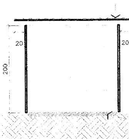
CORTE B ESC: 1:50
