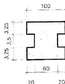
CORTE PILAR ESC: 1:50
