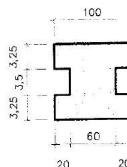
CORTE PILAR ESC: 1:50
