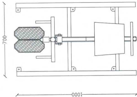
PLANTA BAIXA
