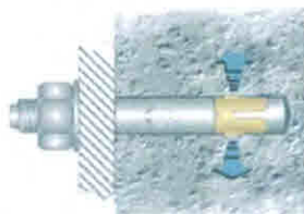
Sistema de Aperto de Chumbadores/Parafusos dentro do Concreto
