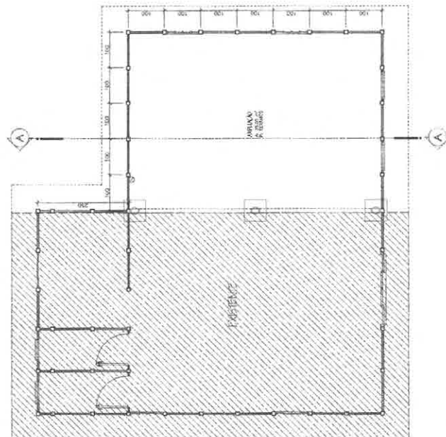
PLANTA BAIXA ENC. 1.50
