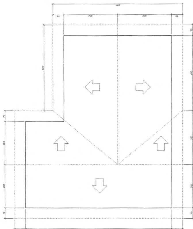
PLANTA DE COBERTURA 1982-1983
