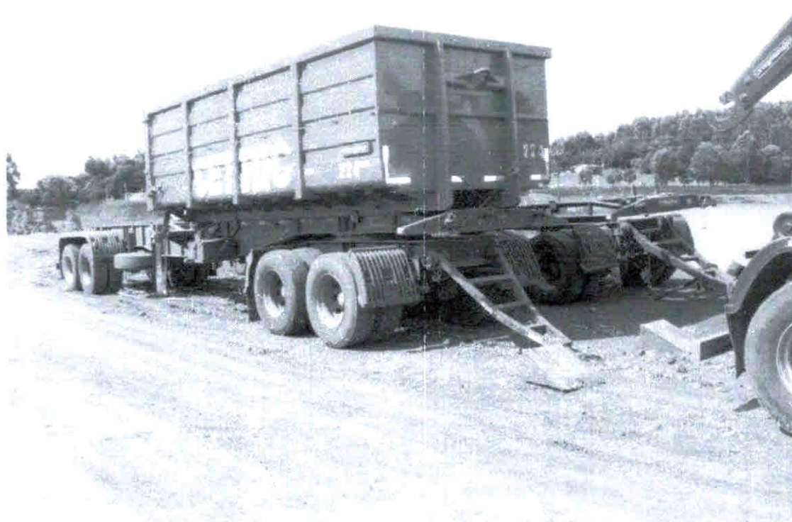
Figura 08 – Contêiner para armazenamento de 25 m 3 .
