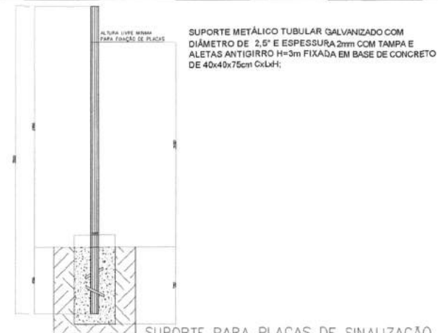
SUPORTE PARA PLACAS DE SINALIZAÇÃO ESCALA: 1:25
