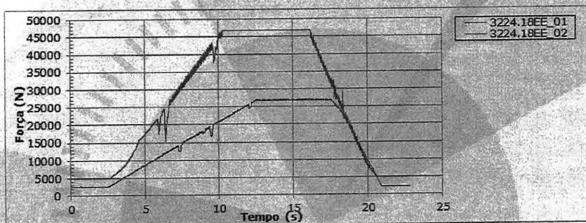
Figura 3: Gráfico Força (N) x Tempo (s).
