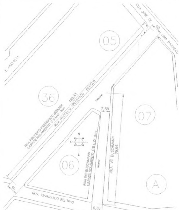
RUA PREFEITO FREDERICO BERGER - PAVIMENTAÇÃO / RECAPE Escala: 1:500
