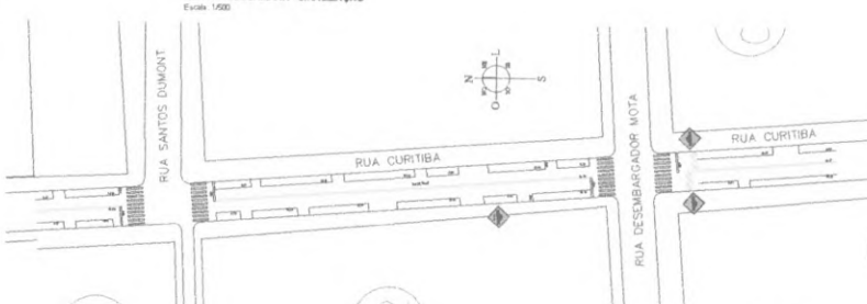
RUA CURITIBA - SINALIZAÇÃO Escala: 1:500
