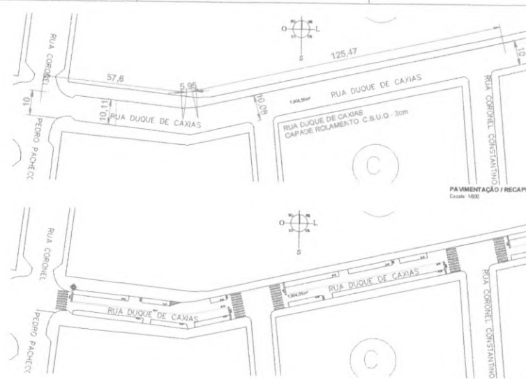
SINALIZAÇÃO Escala: 1:500
