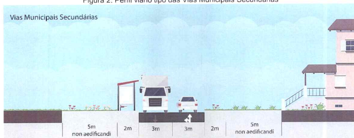
Figura 2. Perfil viário tipo das Vias Municipais Secundárias
