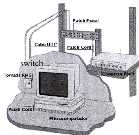
Figura 2 - Componentes de um sistema de cabeamento horizontal
